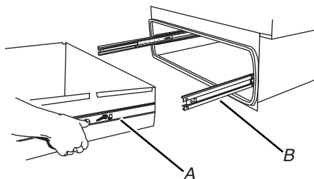
A. Rallo del cajón B. Guía del cajón
