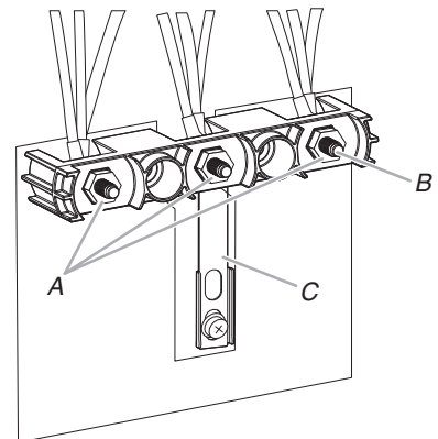
A. Écrou 10-32 à tête hexagonale B. Bornes C. Barrette de liaison à la terre
