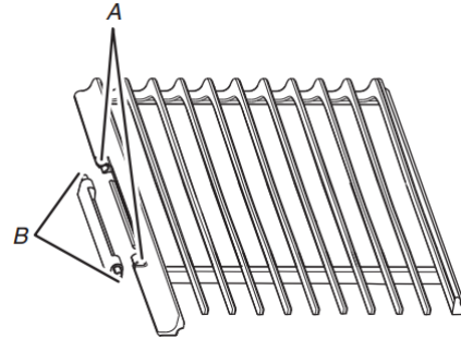
A. Grate slot B. Hinge pin
