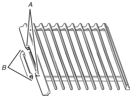
A. Ranura de la rejilla B. Pasador de bisagra
