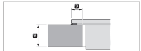
Fig. 11.7 Cote d'appui pour montage en saillie
