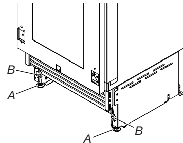
A. Patas niveladoras B. Pernos de ajuste
