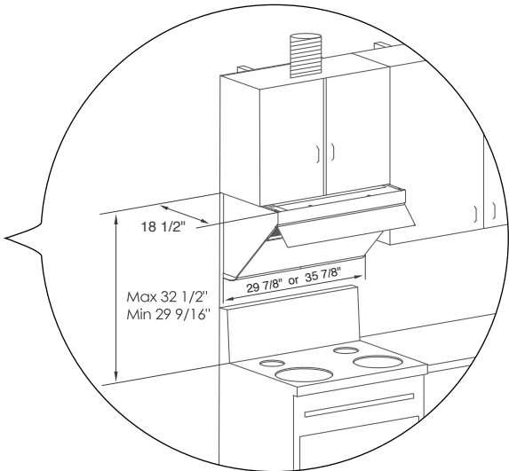
柜下安装
