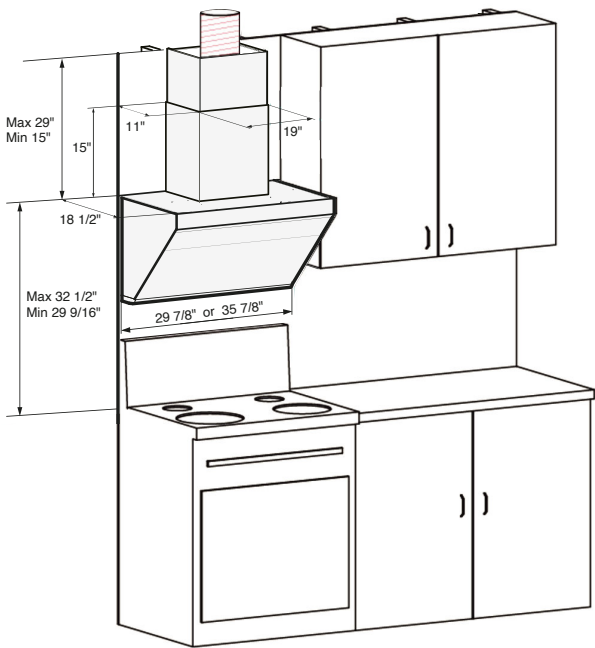
壁挂安装
