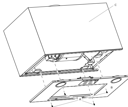
A. 4 vis à tête plate- 3,5 x 9,5 mm B. Plaque avant C. Placard
